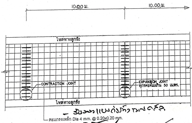
แบบขยาย CONTRACTION JOINT มาตราส่วน NOT TO SCALE
